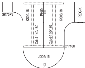
Sestava kanc.stolů na podnoži C1/160 s dělicí příčkou bez políc
