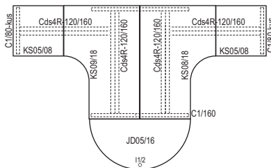
Sestava kanc.stolů na podnoži C1/160 s použitím rohových kanálů a nohou C1/80
