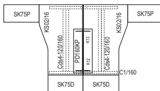
Sestava kanc. stolů na podnoži C1/160
