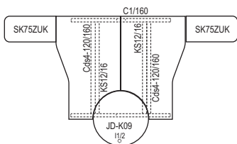
Sestava kanc.stolů s vloženým jednacím kruhem na podnoži C1/160
